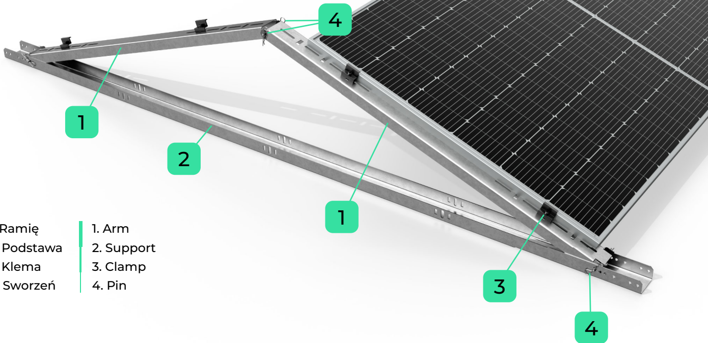
Układ paneli i klemy Modules & clamps layout
