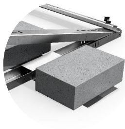
balastowanie ballasting
